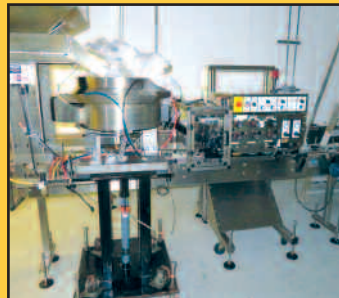
Charleston Hot Fill Puck Inverter
